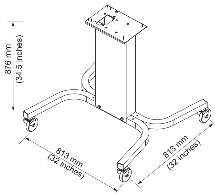
Figura A-5. Soporte de Impresora móvil
